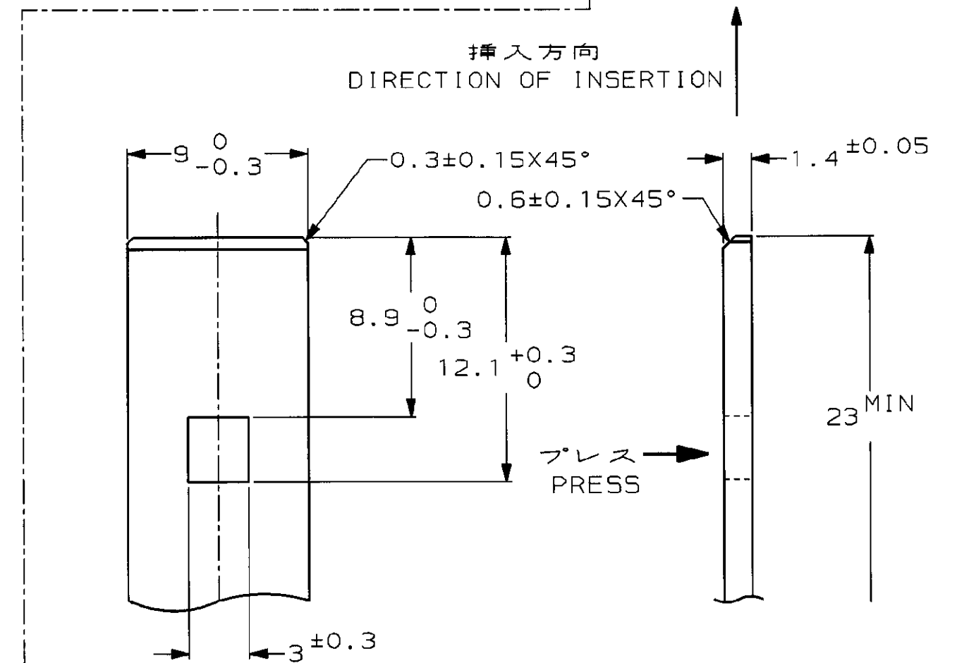
ブラケット推奨寸法 RECOMMENDED DIMENSIONS OF BRACKET SCALE 4 : 1
